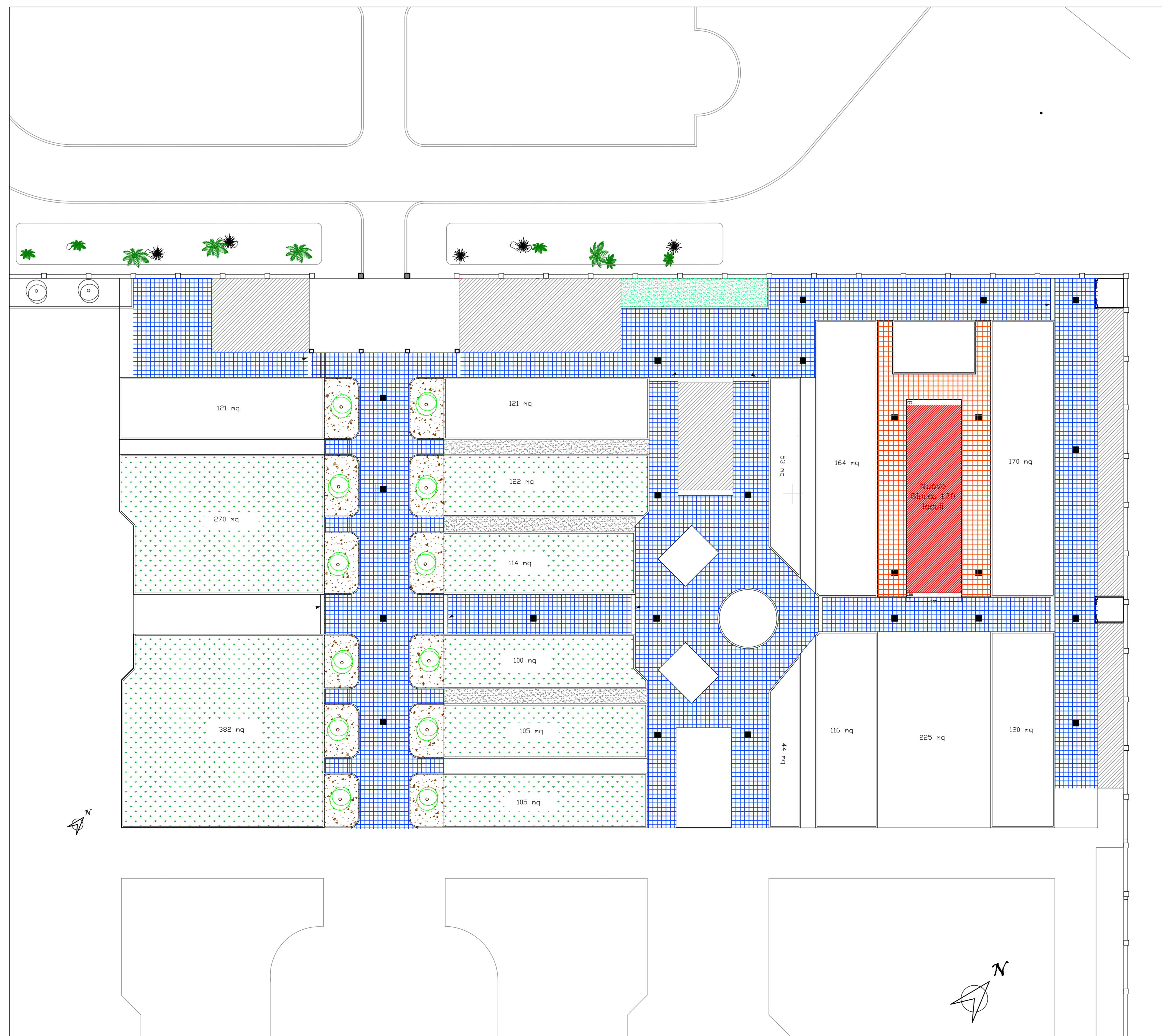
PLANIMETRIA SISTEMAZIONE VIALI NUOVO CIMITERO - PRIMO LOTTO PRIMO STRALCIO - REALIZZAZIONE BLOCCO LOCULI N.3
