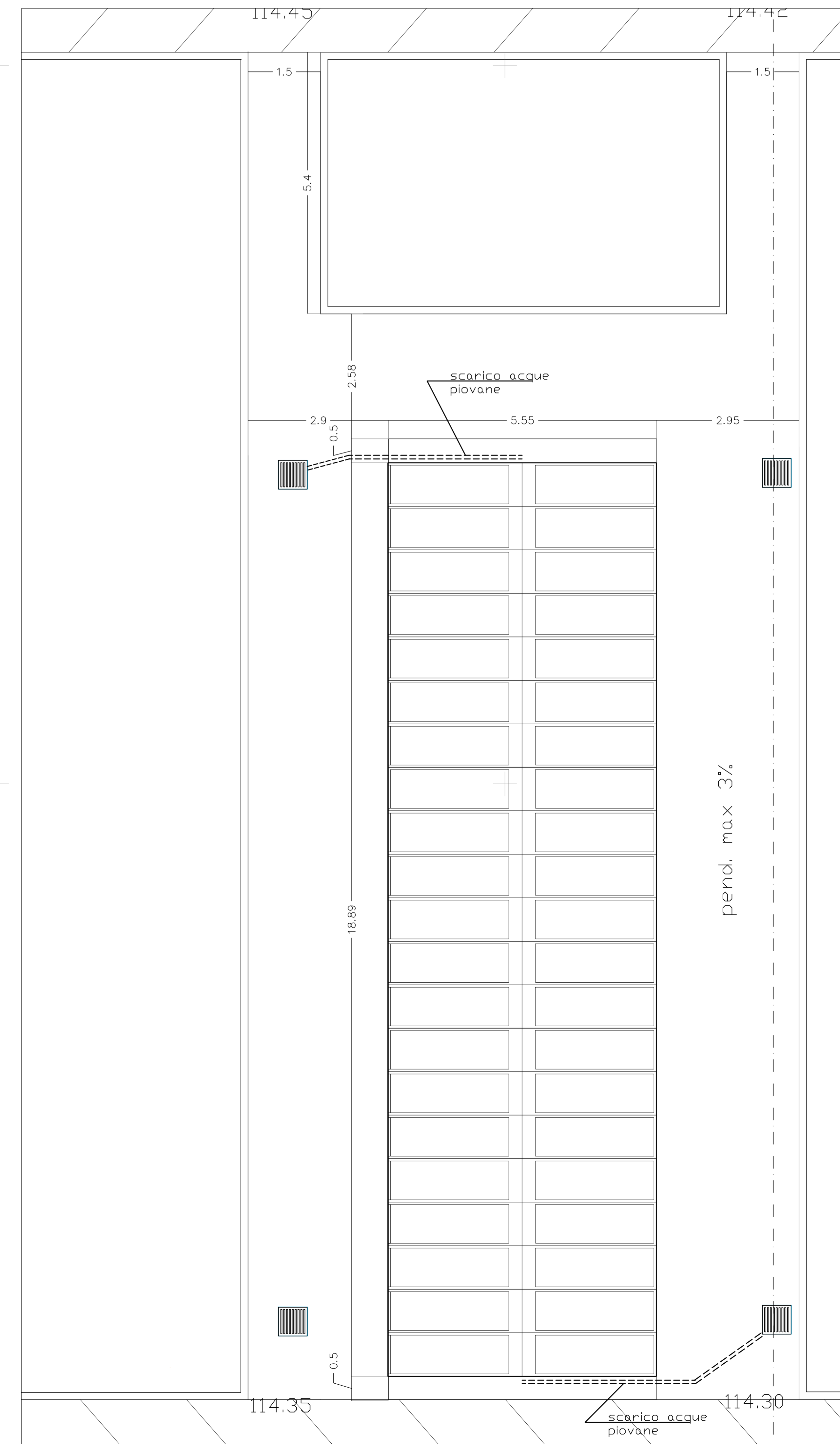
PLANIMETRIA REALIZZAZIONE BLOCCO LOCULI N.3
