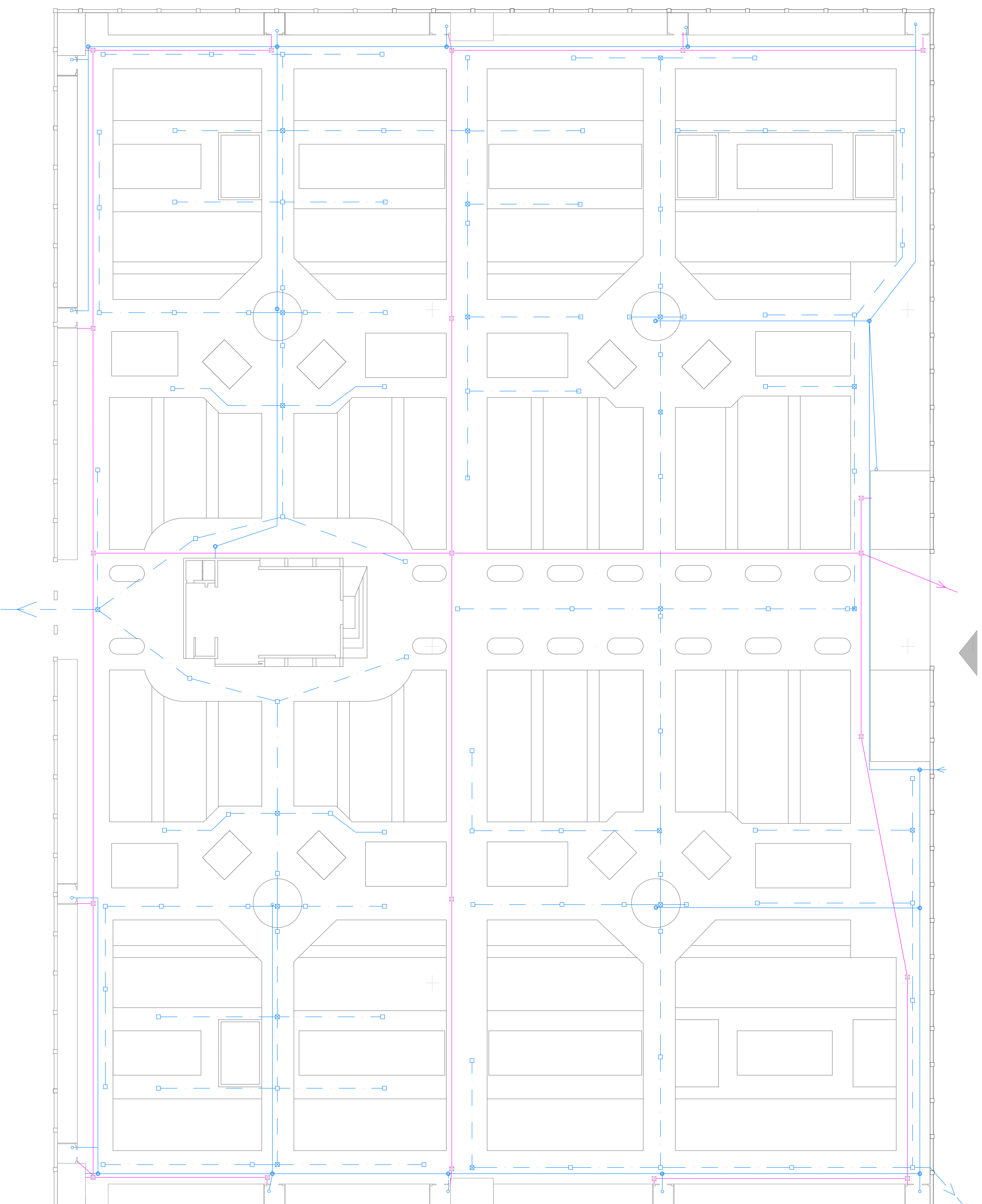
PLANIMETRIA RETI IDRICHE NUOVO CIMITERIO - stato di progetto
